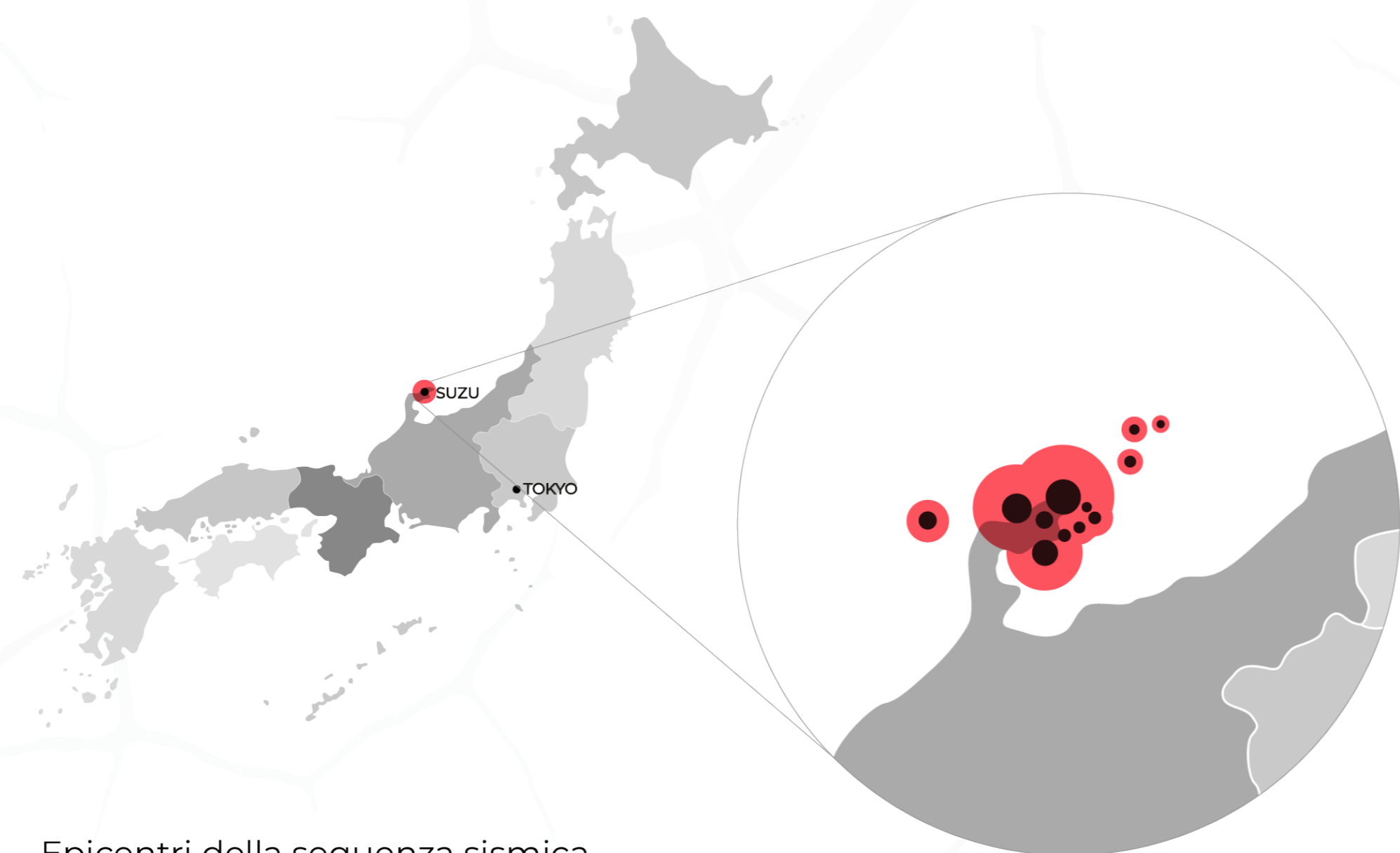
Epicentri della sequenza sismica avvenuta in data 01-01-2024. Credits: Japan Meteorological Agency.
